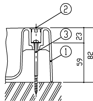
固定部詳細(1/3)
